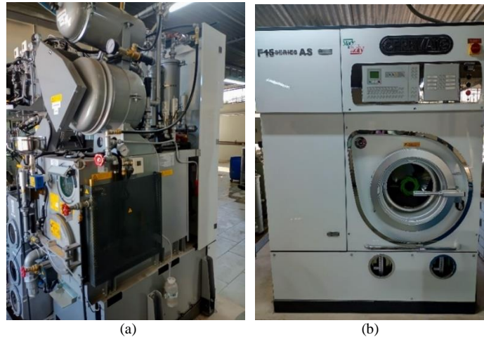
Figura 1. Lavadora en seco multisolvente. (a)Vista lateral-posterior (b)Vista frontal Fuente. Registros internos Reactivos Jeans S.R.L.
